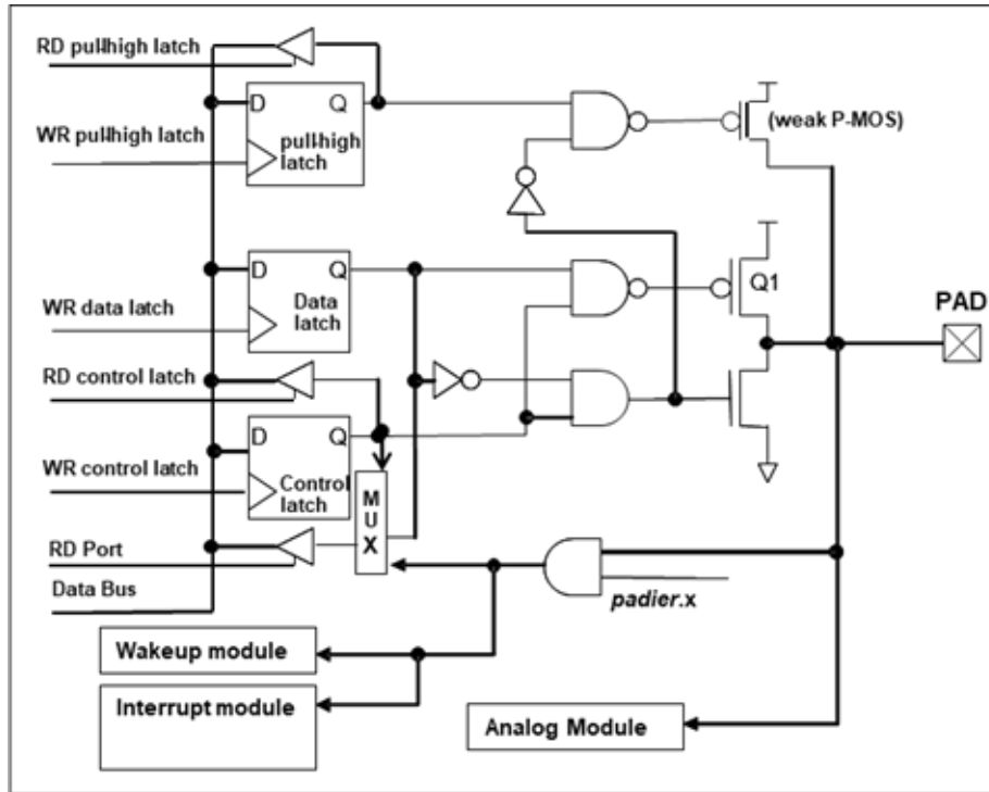
图.15: IO 引脚缓冲区硬件图
