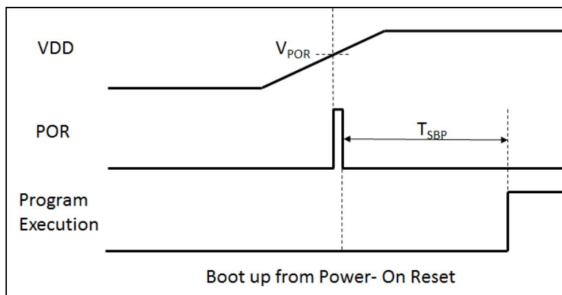
图.1: 上电时序
