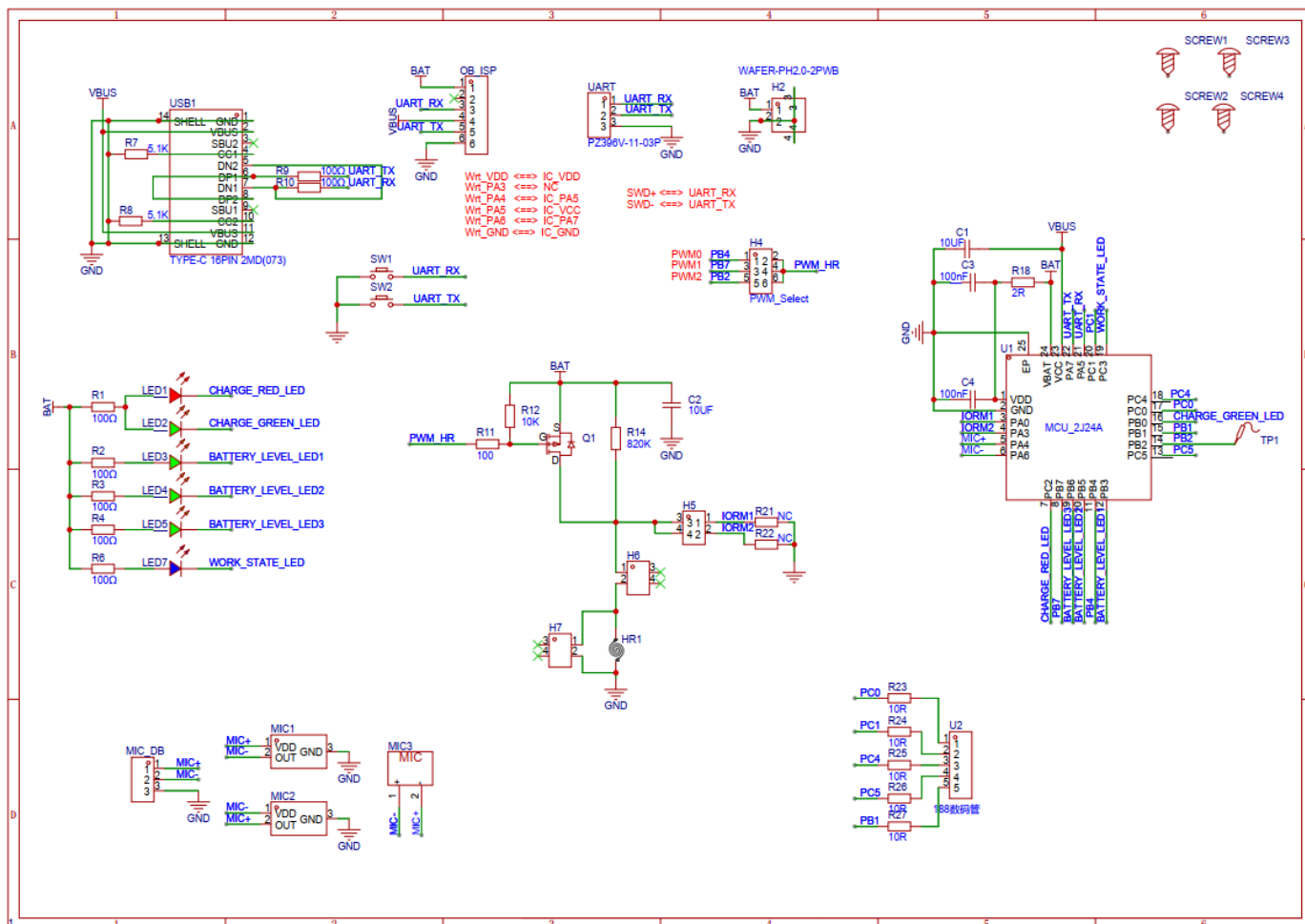
图.22: DemoBoard 原理图
